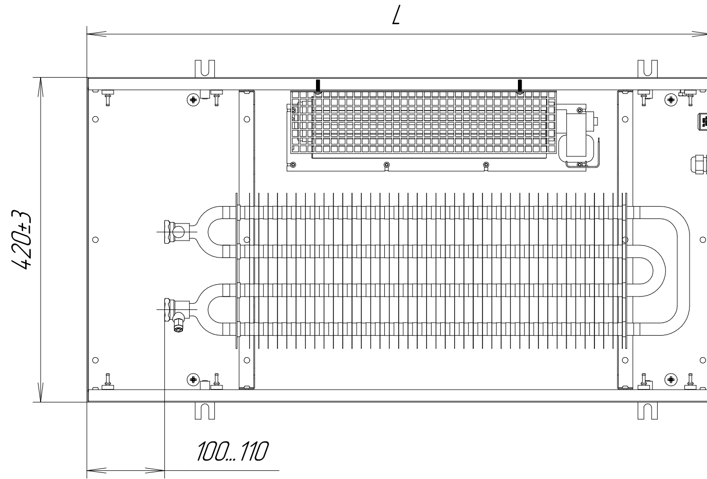
KVPV 420-120-L.00.000
