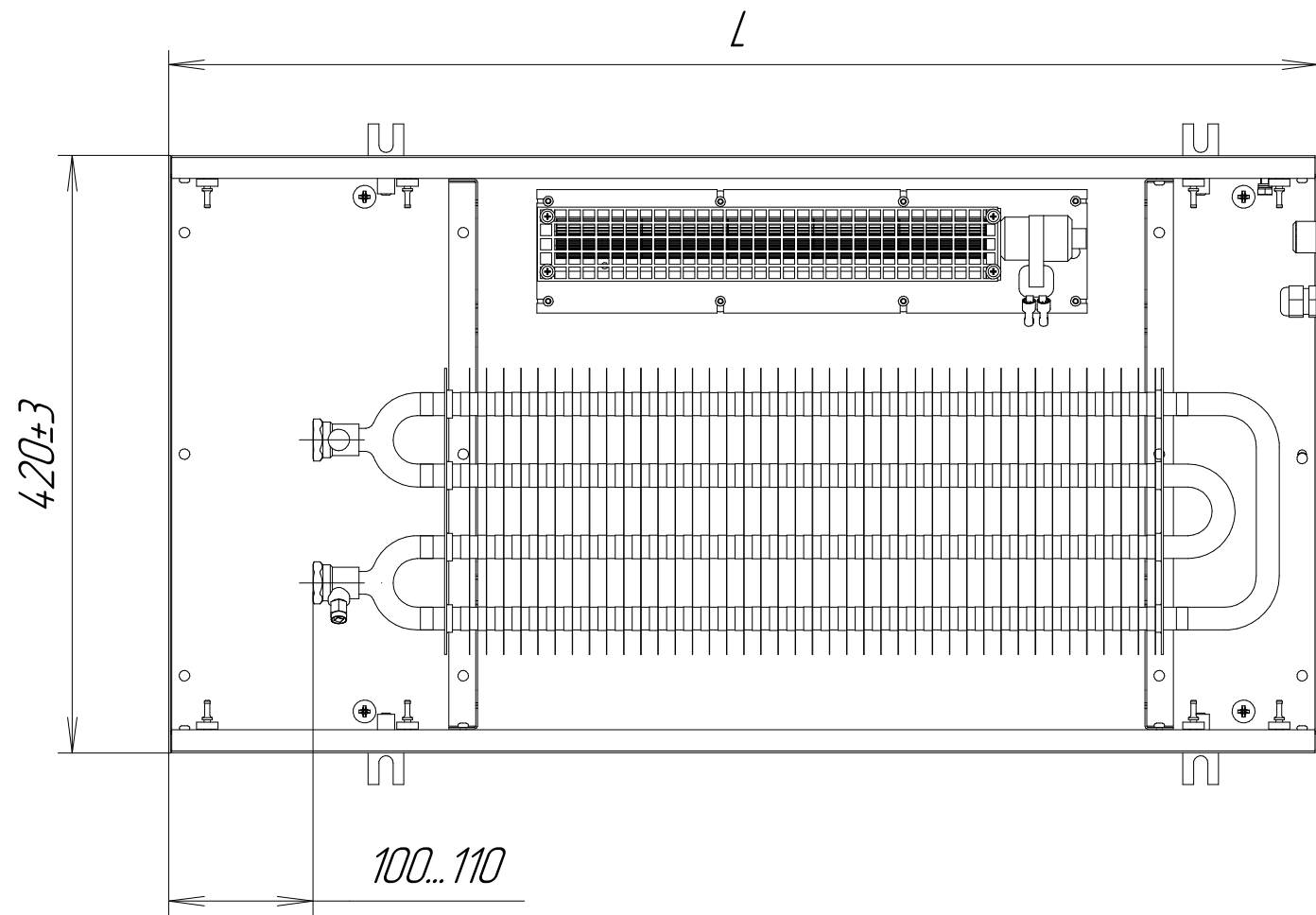
KVPV 420-85 (-105)-L.00.000
