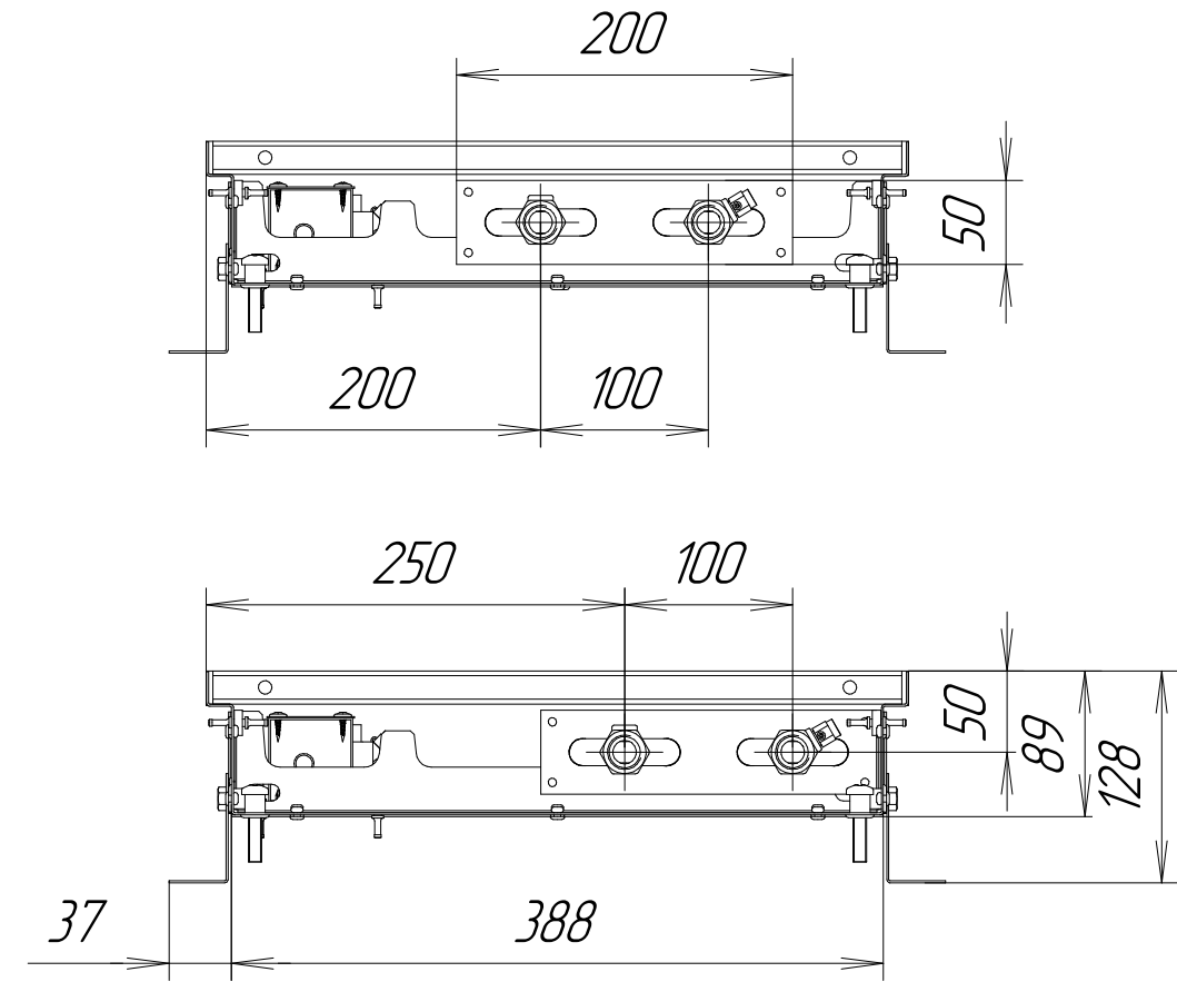
KVZV (KVPV) 420-85-L.00.000
