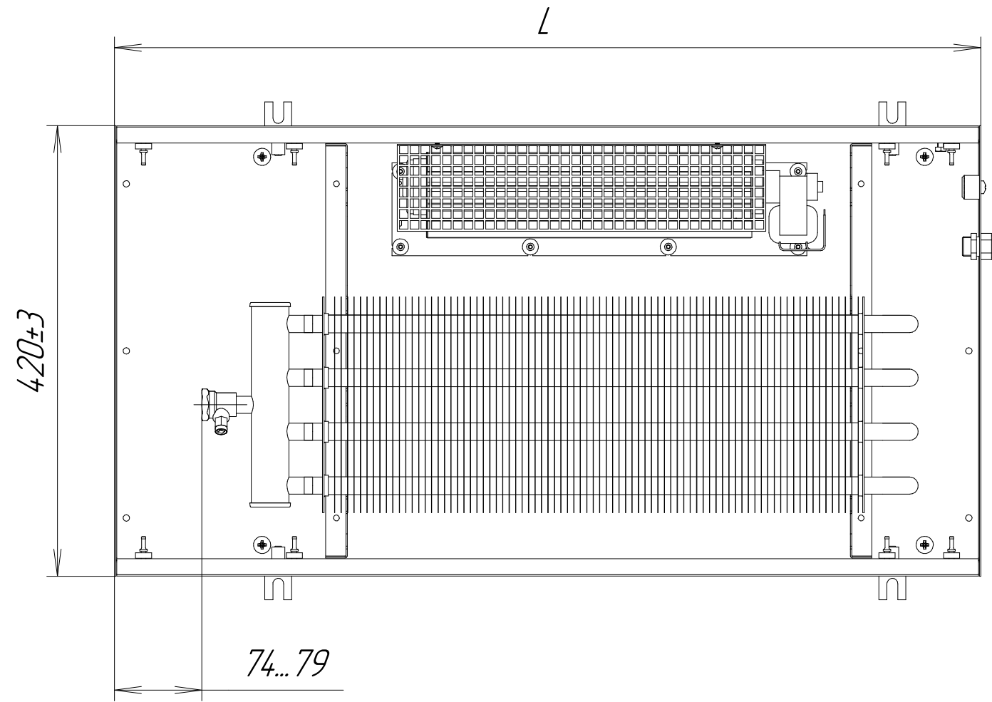
KVPV 420-140-L.00.000
