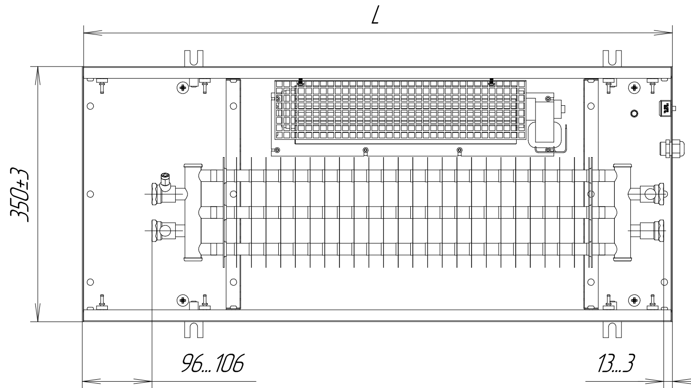
KVPV 350-140-L.00.000
