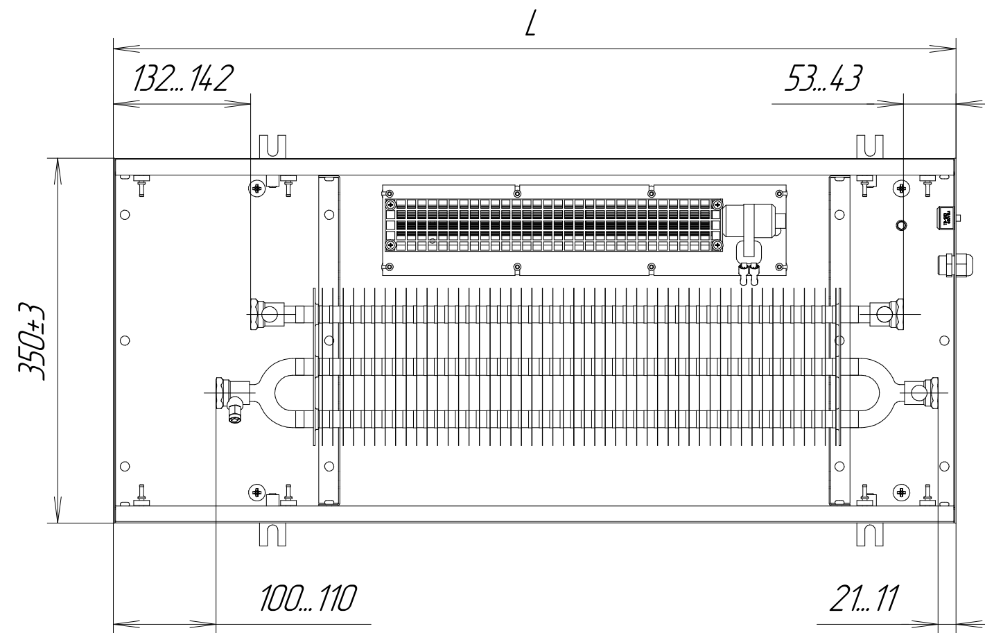
KVPV 350-85 (-105)-L.00.000
