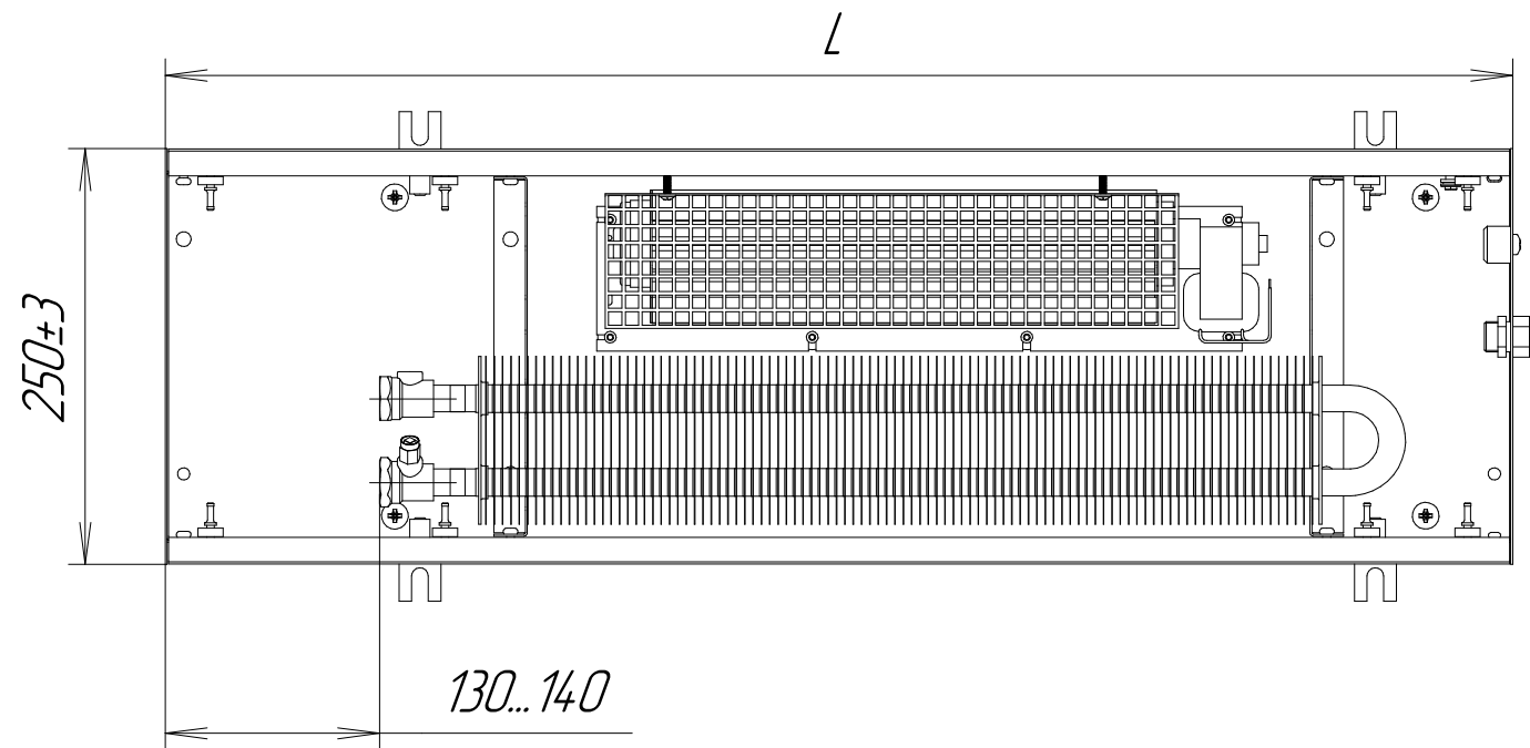
KVZV 250-120-L.00.000
