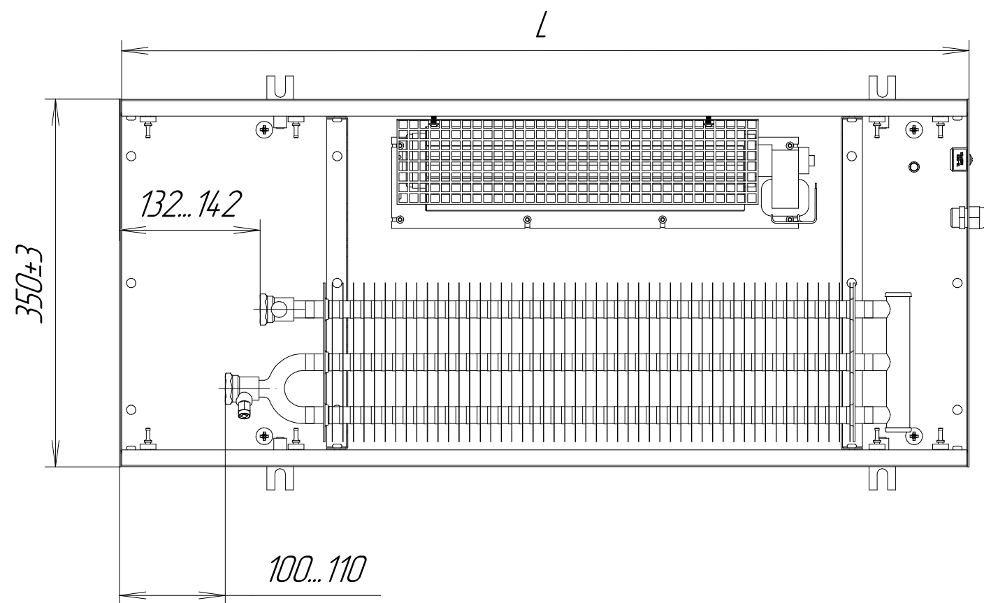
KVPV 350-120-L.00.000
