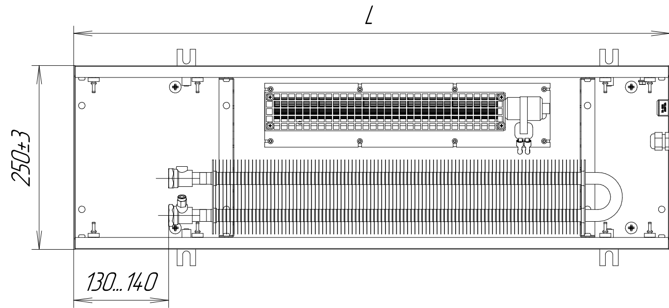
KVPV 250-85 (105)-L.00.000
