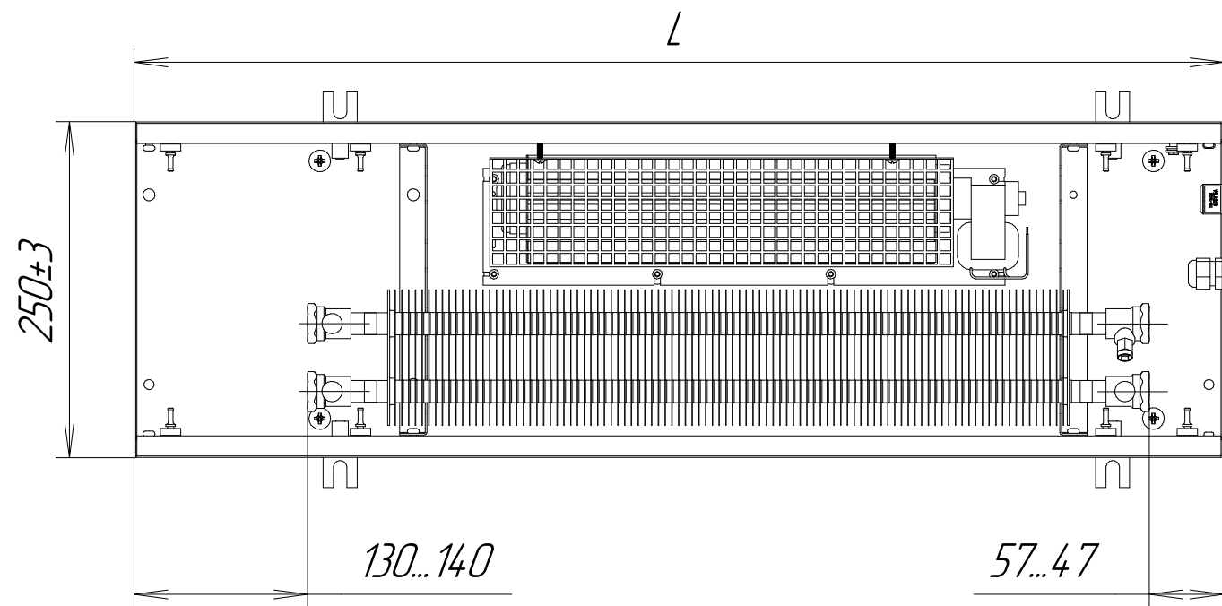
KVPV 250-120-L.00.000
