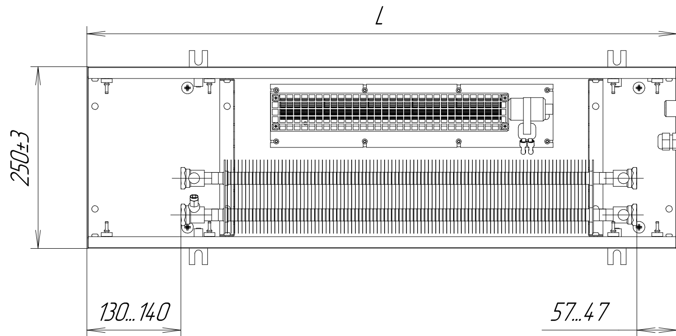
KVPV 250-85 (105)-L.00.000
