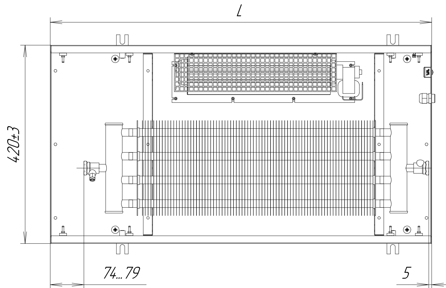
KVPV 420-140-L.00.000
