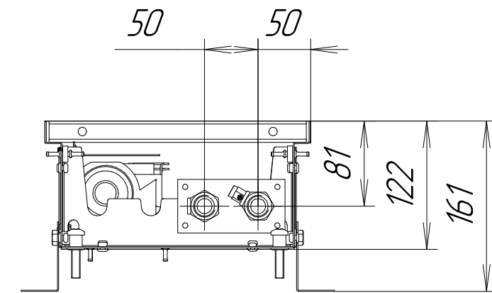
KVZV (KVPV) 250-120-L.00.000
