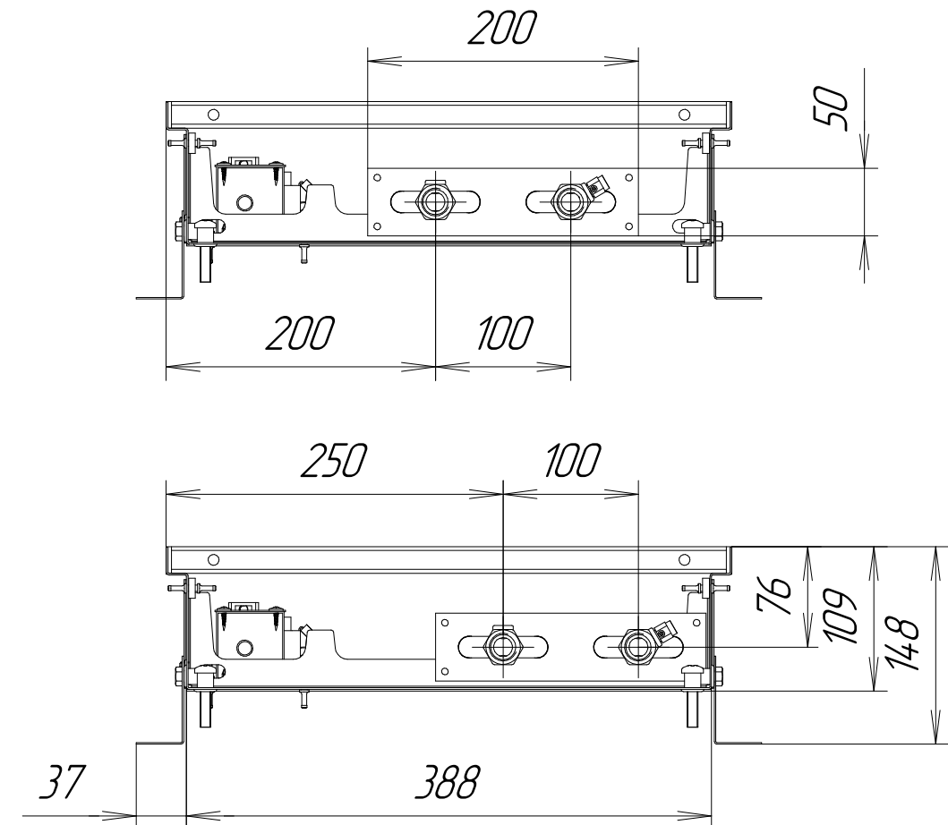
KVZV (KVPV) 420-105-L.00.000
