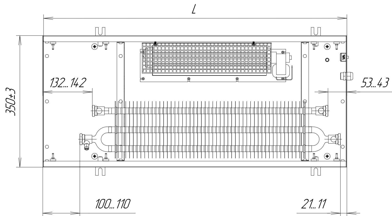
KVPV 350-120-L.00.000
