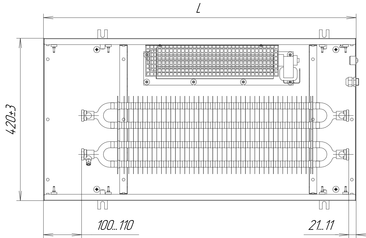
KVPV 420-120-L.00.000
