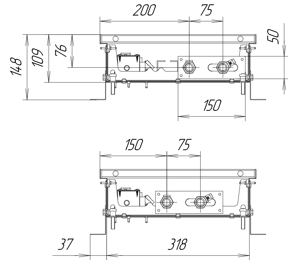
KVZV (KVPV) 350-105-L.00.000
