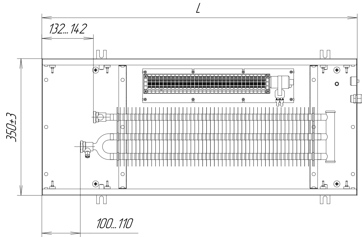
KVZV 350-85 (-105)-L.00.000
