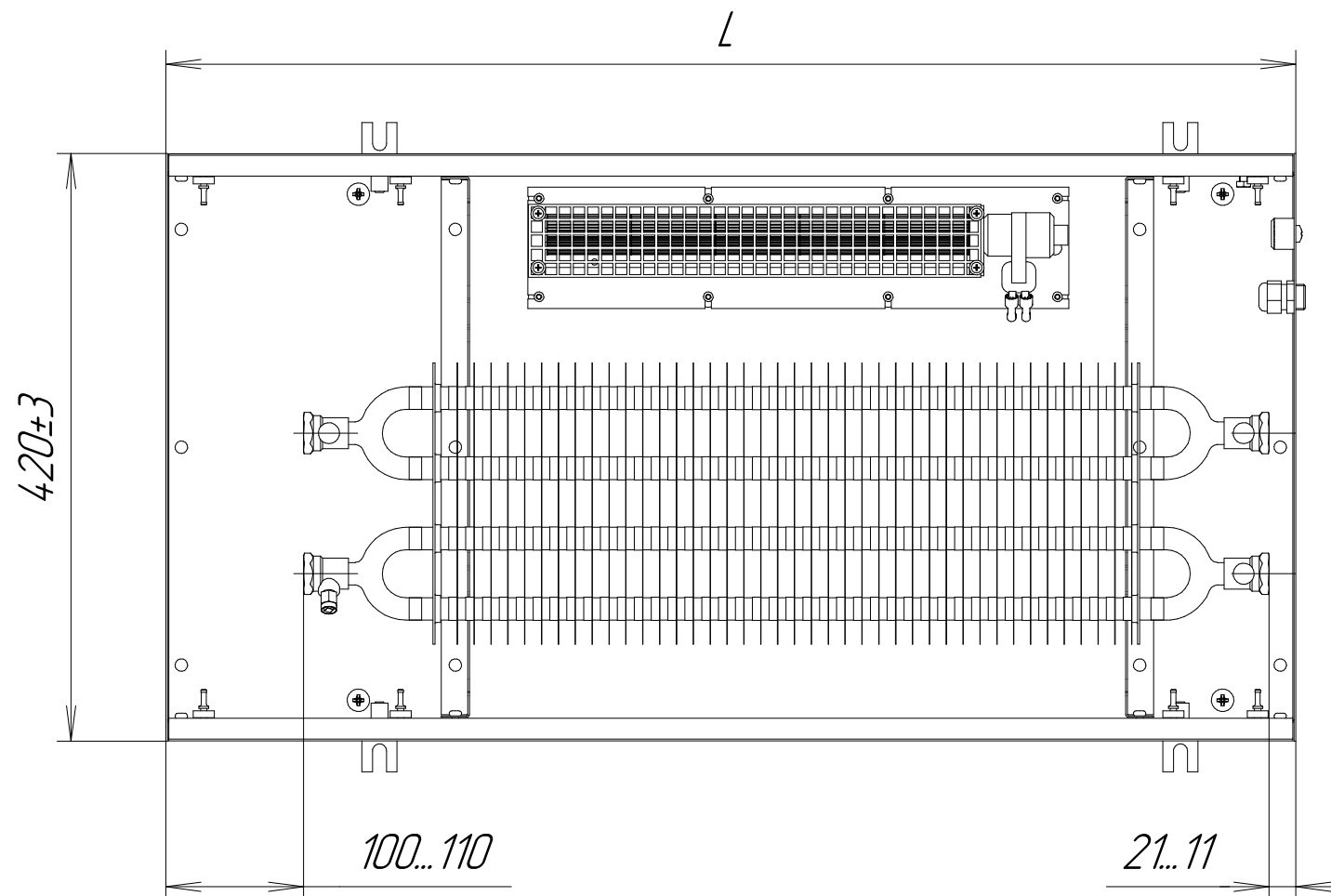
KVPV 420-85 (-105)-L.00.000
