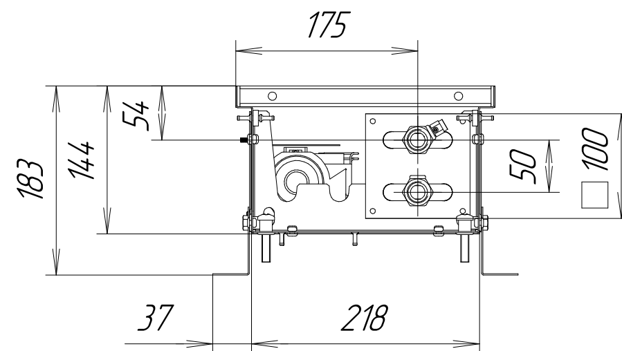
KVZV (KVPV) 250-140-L.00.000
