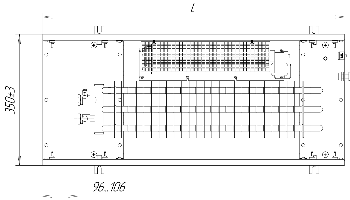
KVPV 350-140-L.00.000
